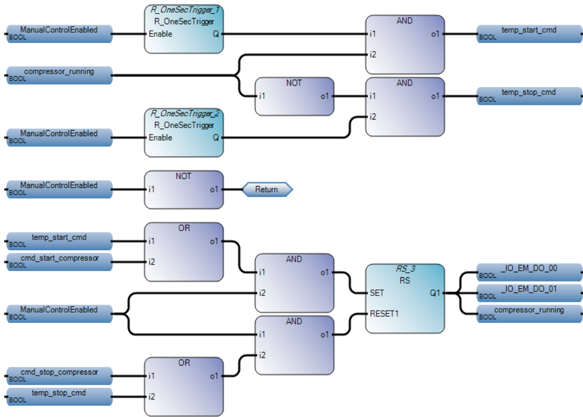
Figure 34. ManualCompressorControl FBD
