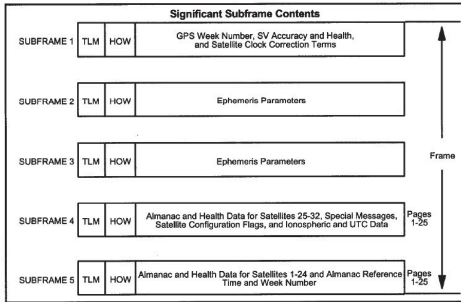
Figure 9. GPS Navigation Message Content [28]
