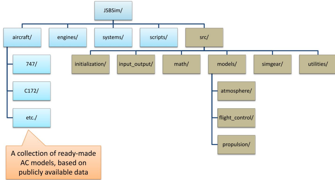
Figure 17. JSBSim Directory Structure [23]
