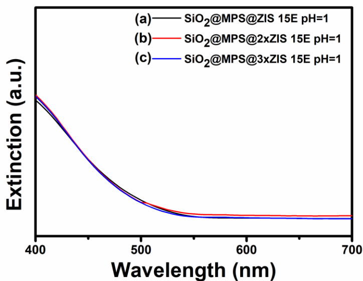
Figure 16. UV spectra of SiO 2 @MPS@ZIS/2xZIS/3xZIS 15E pH=1
