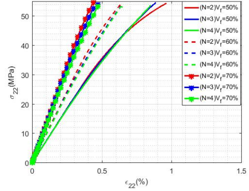
(d) S-2-glass - SC-15 epoxy for N=2,3,4
