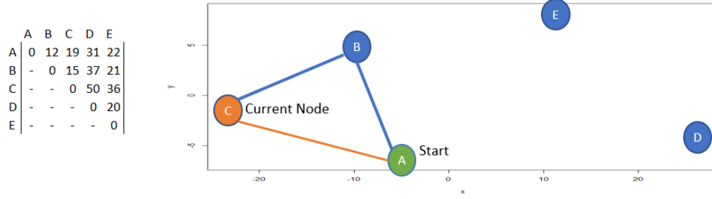
Figure 8. EL Subtour 1
