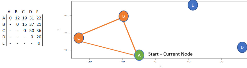
Figure 10. EL Subtour 3
