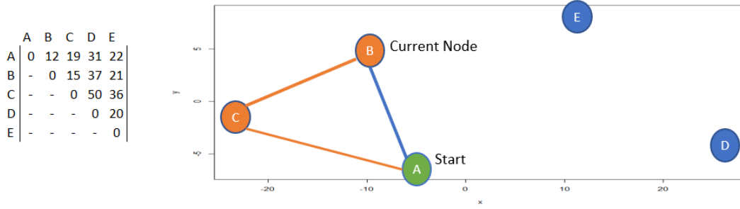
Figure 9. EL Subtour 2
