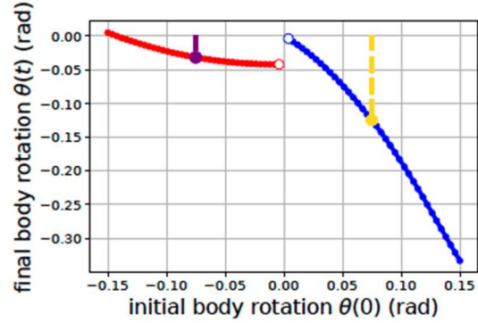
(d) liftoff trajectory outcomes
