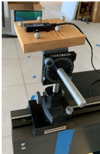
Figure 16. OptiTrack sled
