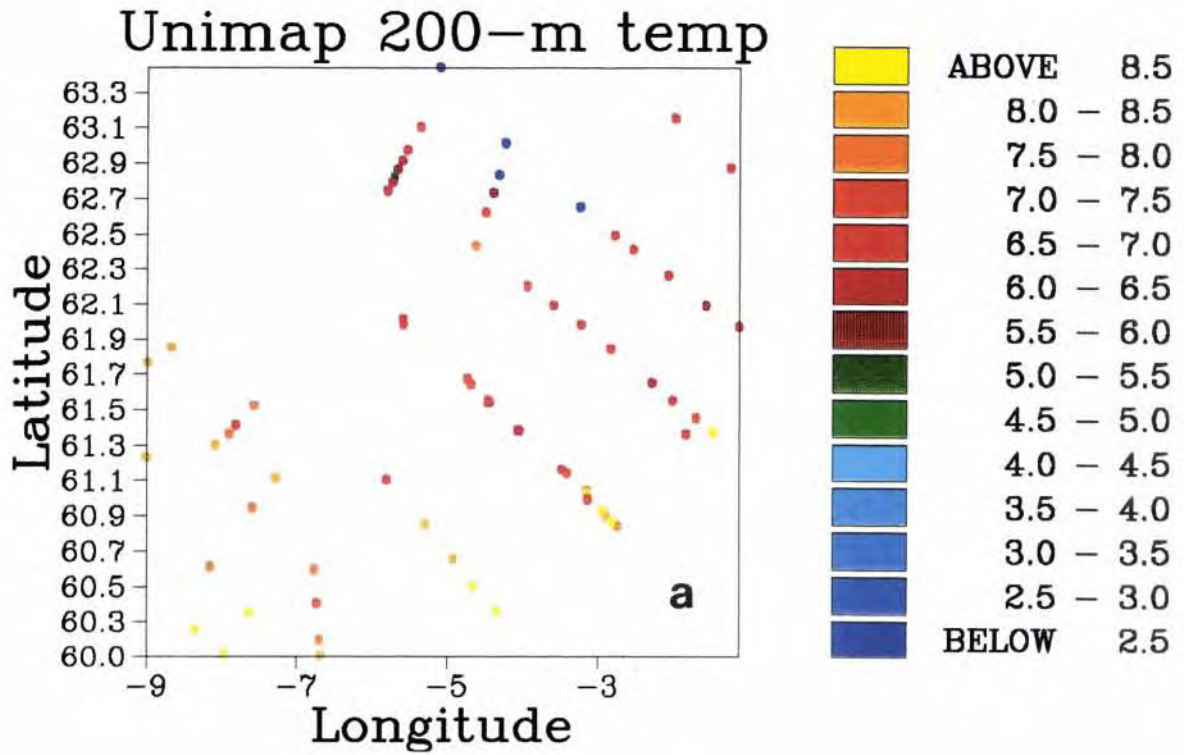
GIN SEA LEVITUS CLIM 200 MET
