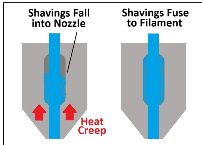
Fig. 17 Shard fusion
