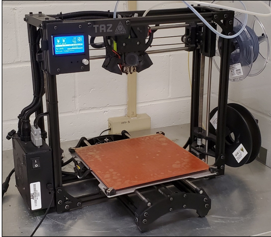
Fig. 1 LulzBot TAZ 5
