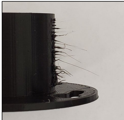
Fig. 6 Webbing
