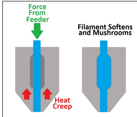
Fig. 16 Heat creep
