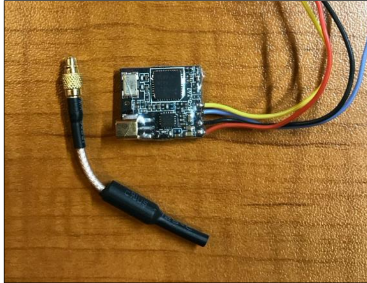
Figure 27. Holybro Atlatl Mini 5.8GHz Video Transmitter.
