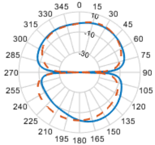
(d) GS at 6.28 GHz.
