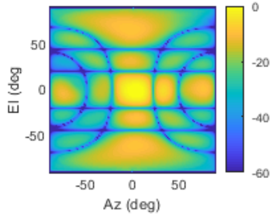
(d) 3 x 3 GS embedded unit cell.
