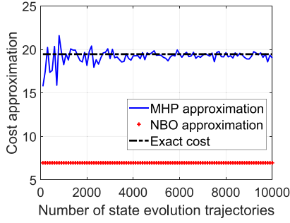
Fig. 3. LQG problem: RS-MHP vs. NBO.
