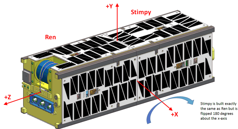
Fig. 4—TEPCE Layout
