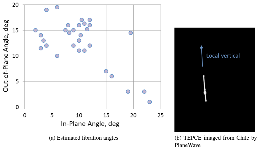
Fig. 33—Tether libration
