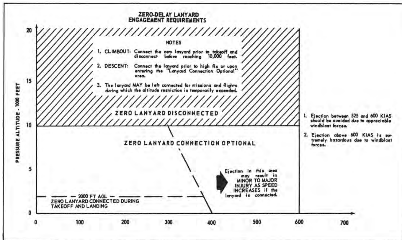
Figure 16-6. Velocity-KIAS.
