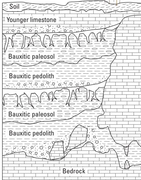
A. Karst bauxite deposits
