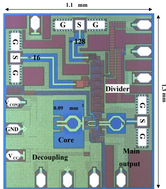
Fig. 6.12. VCO Chip Micrograph
