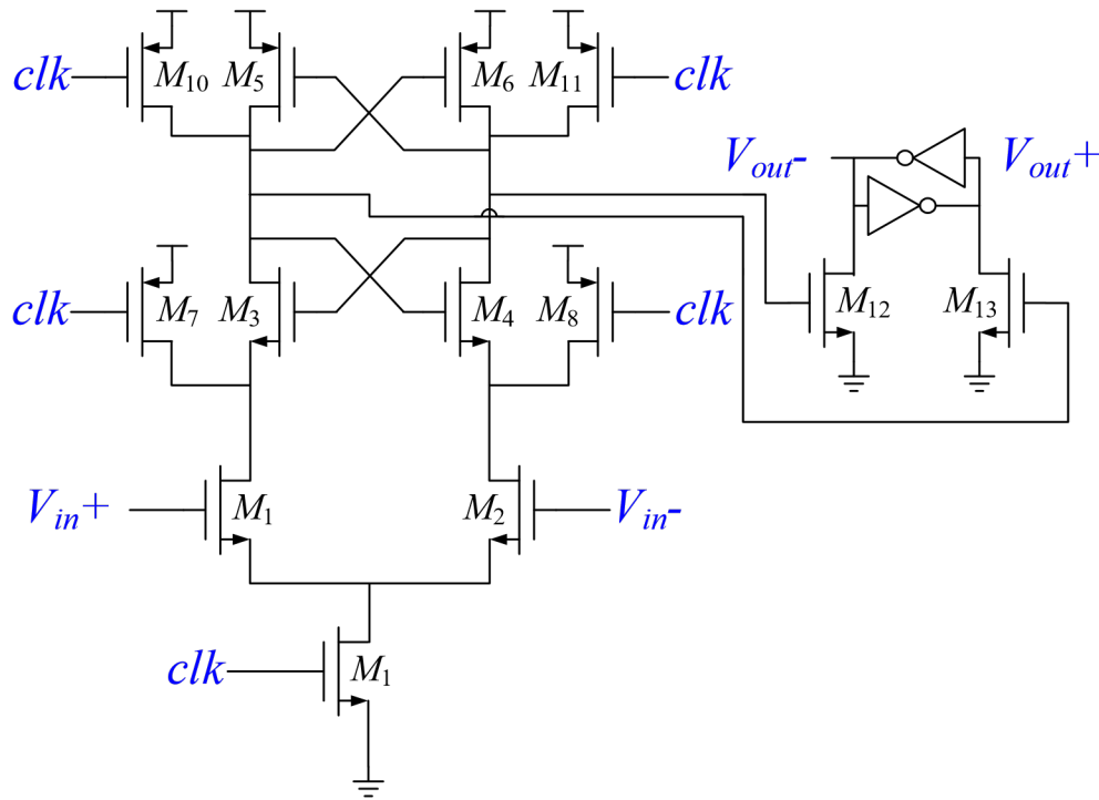
Fig. 7.22. StrongARM Latch
