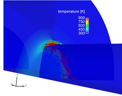
(d) temperature, 10\times vel
