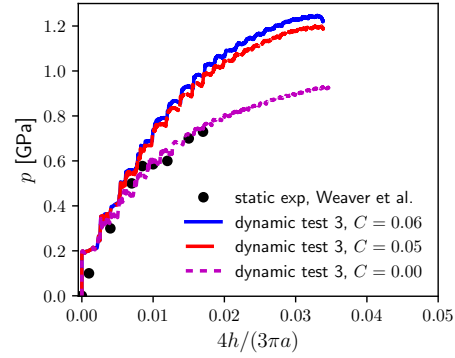
(d) indentation stress-strain
