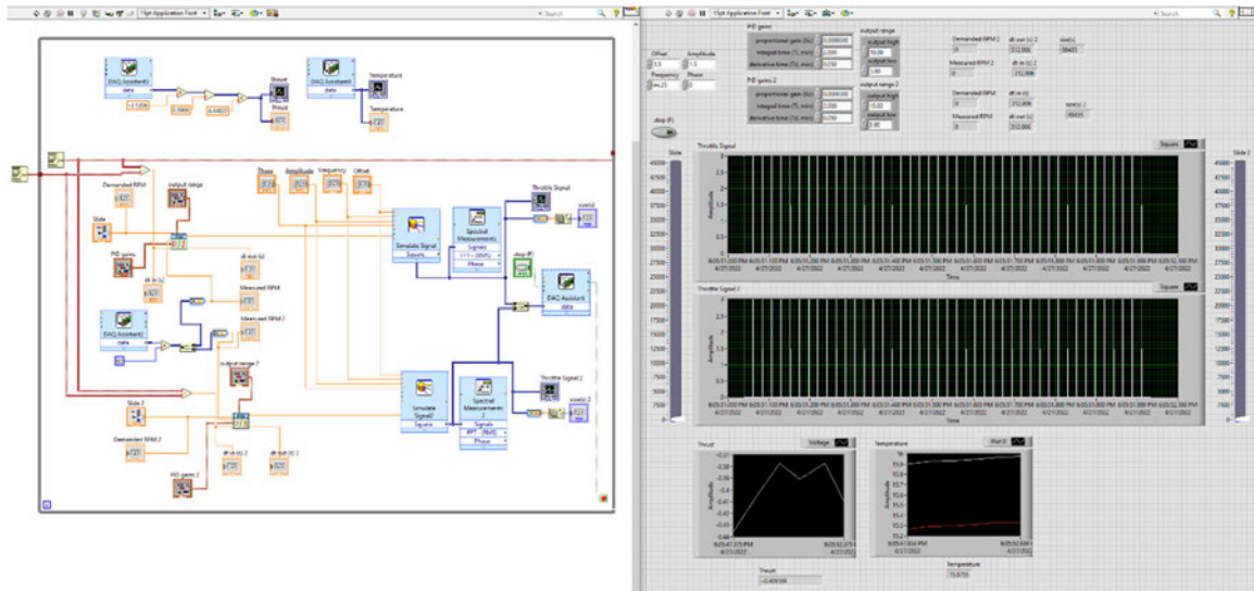
Figure 10. LabVIEW VI.
