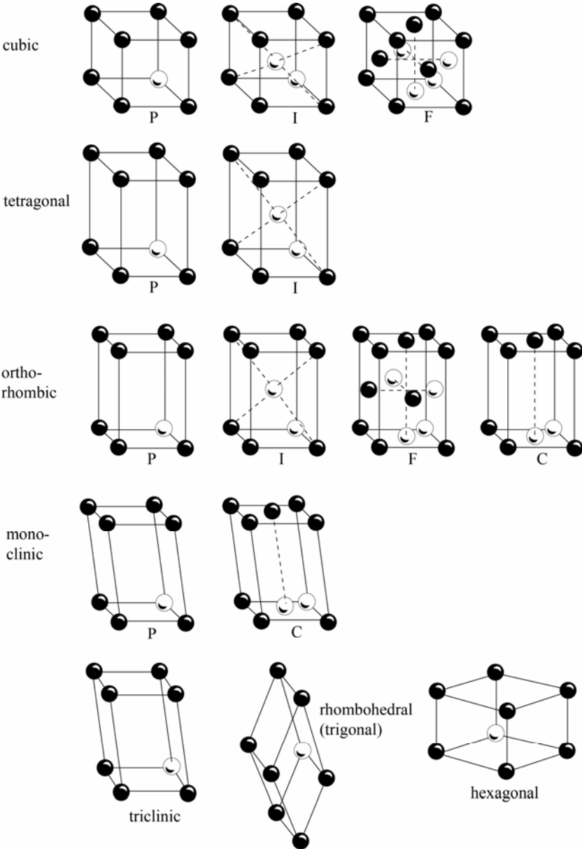
Fig. 3.2 Bravais lattices
