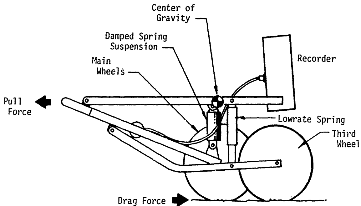
Elevation
