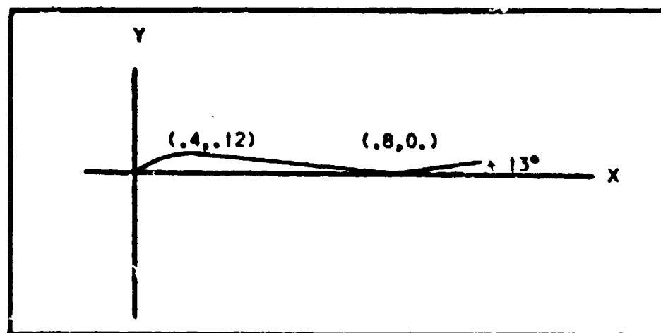
Fig. 4 Reflexed Airfoil
