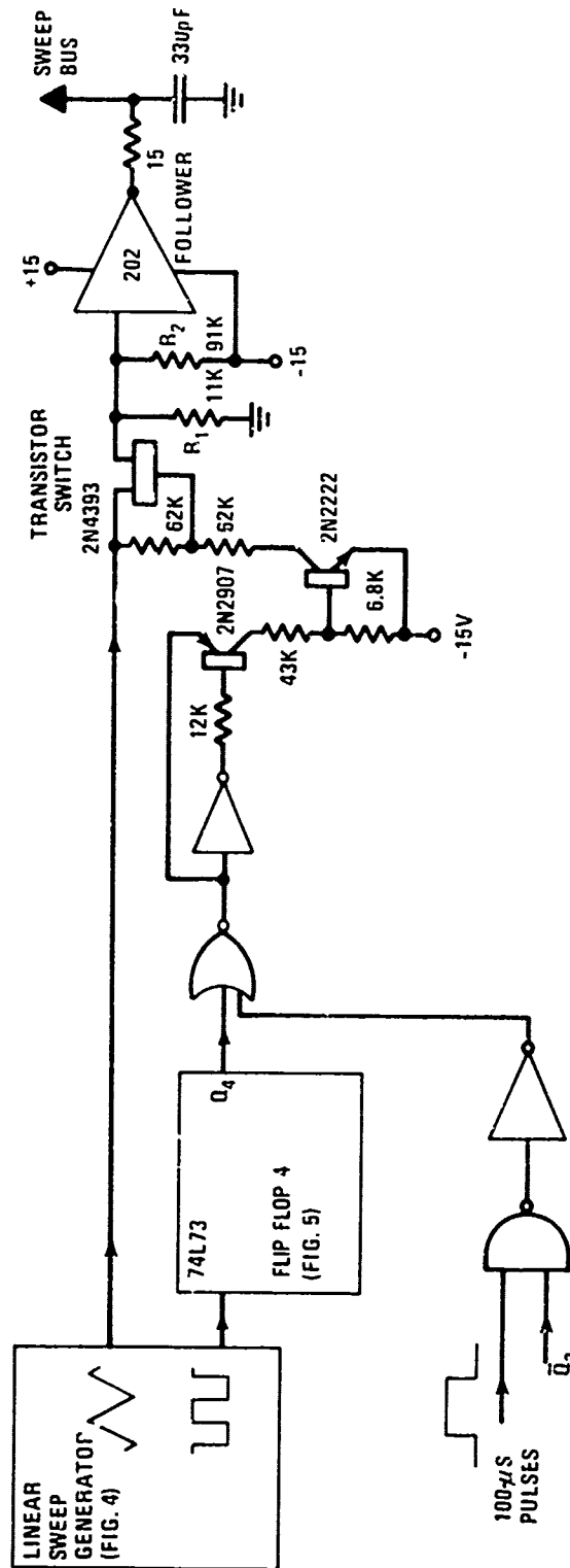
Fig. 6 — Sweep modulator
