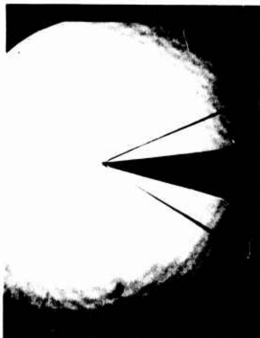
(d) SHADOWGRAPH AT \alpha = +4^\circ
