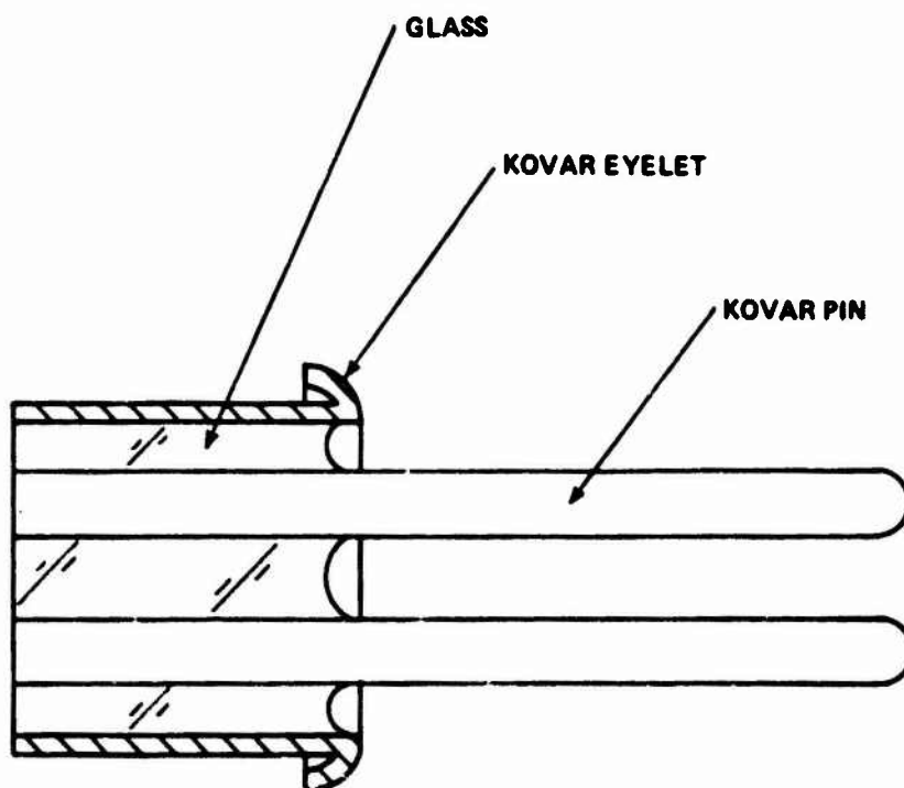
FIG. 1 INITIATOR PLUG
