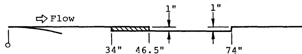
(d) 27.5-inch long shallow-cavity model
