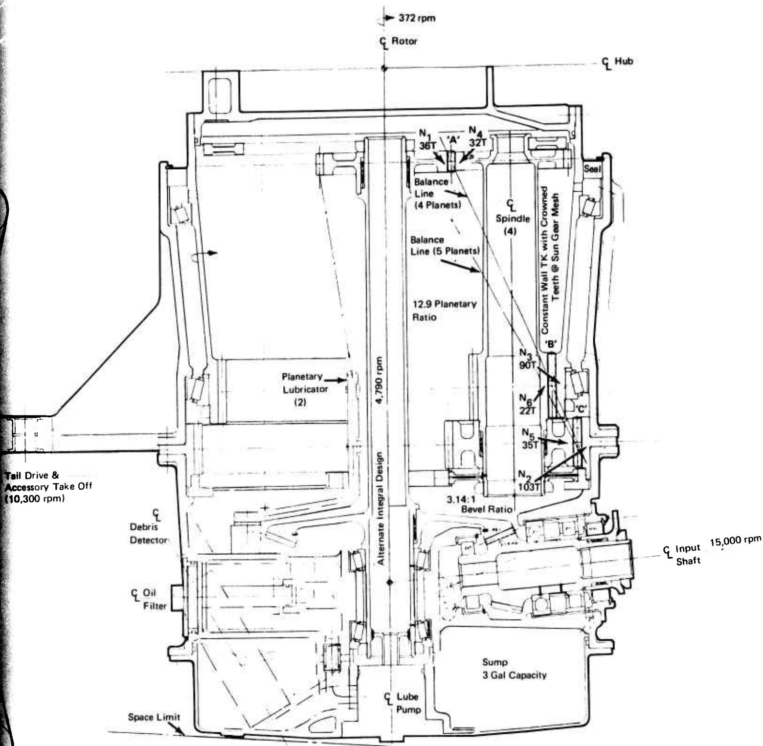
SECTION A-A
