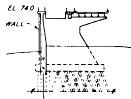
SECTION D-D
