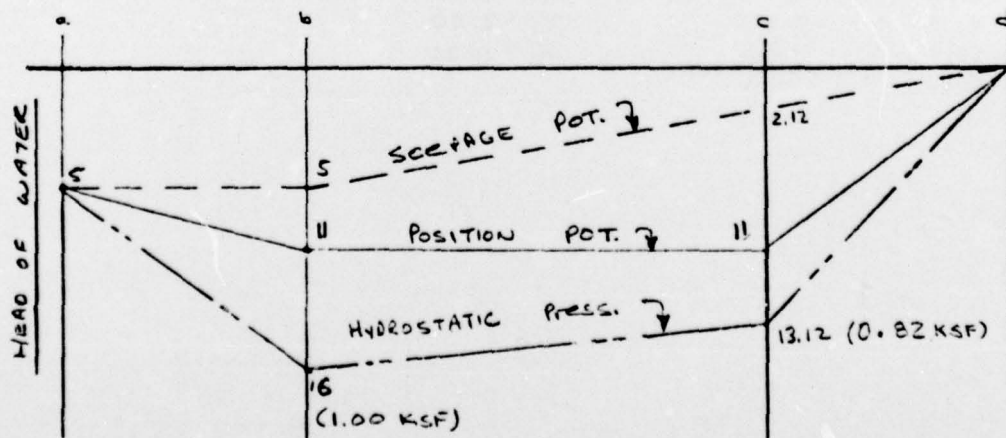
CREEP DIAGRAM
