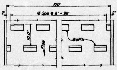
SECTION B-B SCALE: 1/4" = 1'-0"
