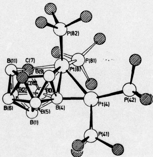
Molecular structure of nido-μ(4,8)-[(Me 3 P) 2 Pt]-8,8-(Me 3 P) 2 -7,8,10-CPtCB 8 H 10 .
