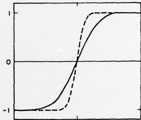
(d) R=3.5, J=0.1
