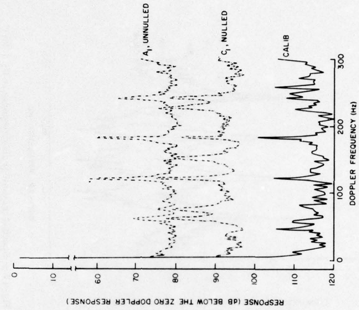
(b) Module 47m
