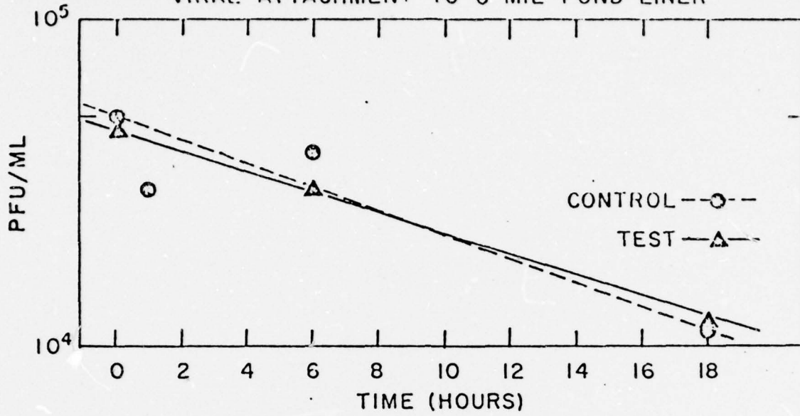
a. GOVALLE FINAL EFFLUENT + POLIOVIRUS
