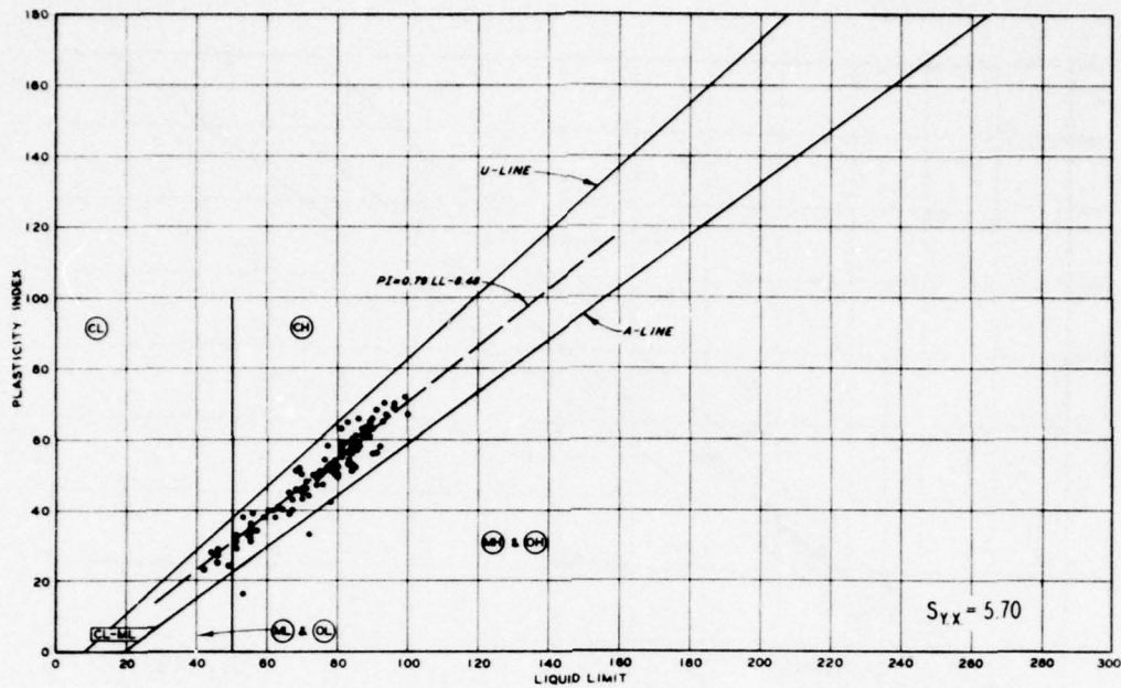
a. Prodelta
