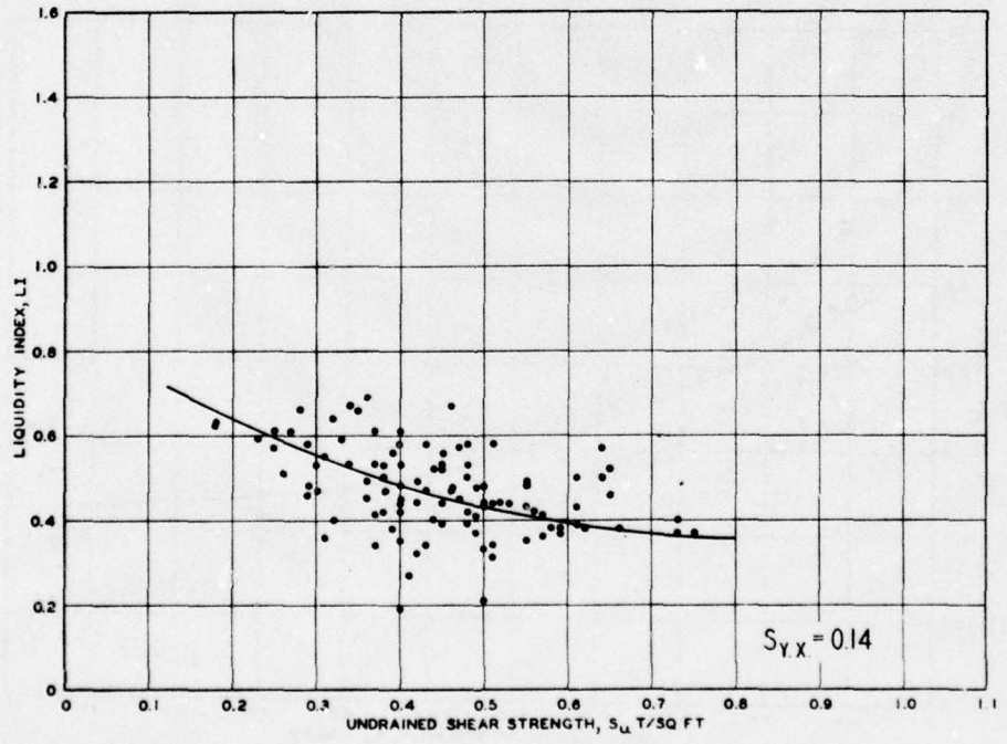
b. Prodelta
