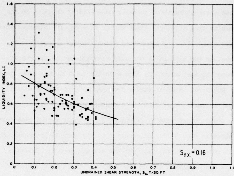
a. Intradelta
