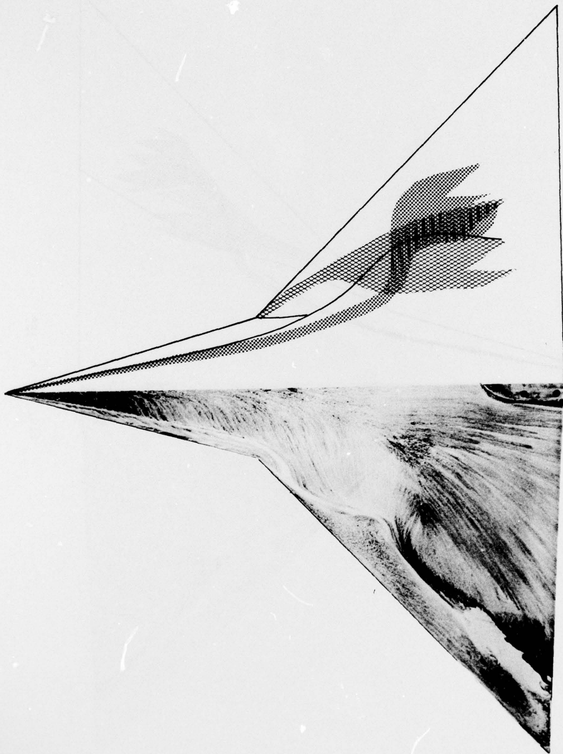
FIG. 14d \alpha = 20^\circ
