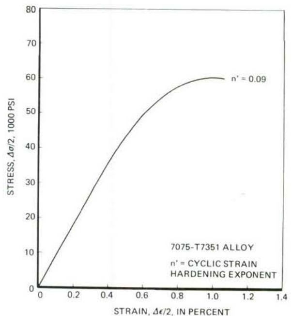
(d) 7075-T7351
