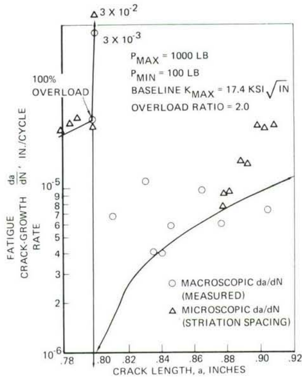
(b) 2024-T8
