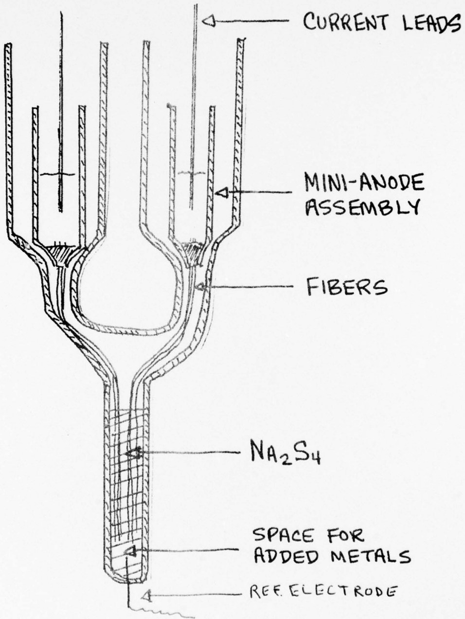
DI ANODE ASSEMBLY
