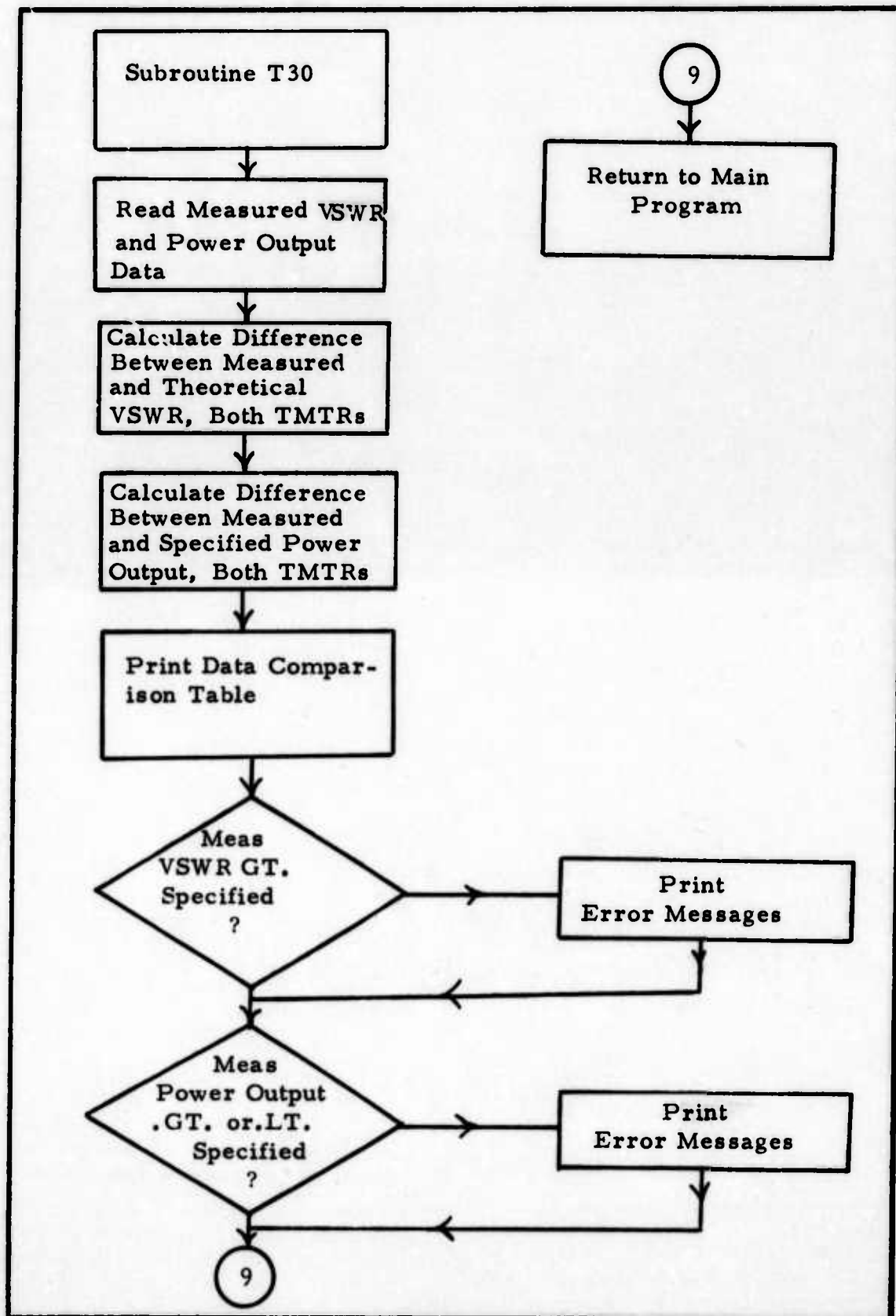
Fig. 17. SUBROUTINE T30
