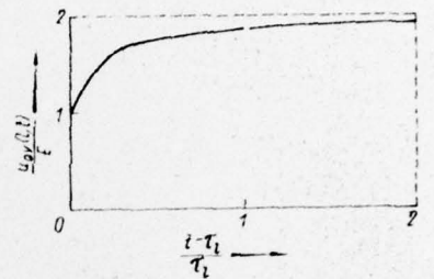
Bild 6. Qualitativer Verlauf der Ausgangsspannung des Koaxialkabels bei Berücksichtigung der Querverluste und Vernachlässigung der Längsverluste
