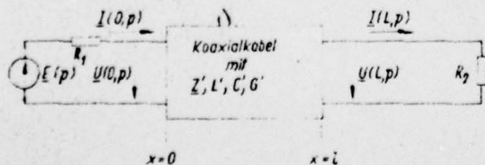
Bild 2. Leitung als Verbindungselement zwischen Spannungsquelle und Abschlusswiderstand
