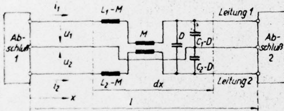
Bild 1. Leitungssystem, Abschlüsse
