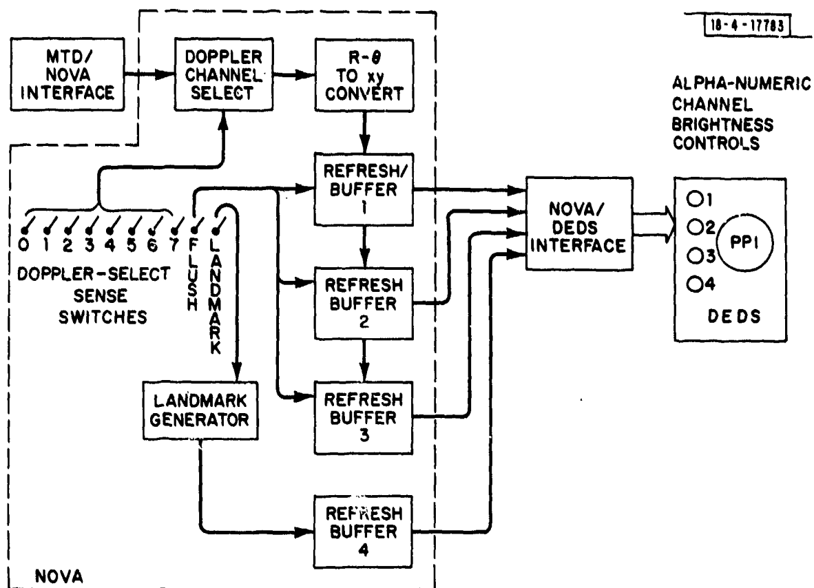
Fig. IV-9. NOVA-DEDS display subsystem.
