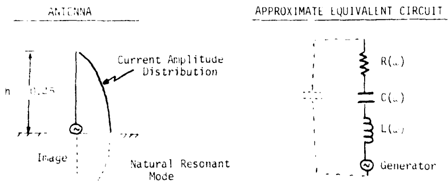
Fig. 1a. Resonant monopole antenna.
