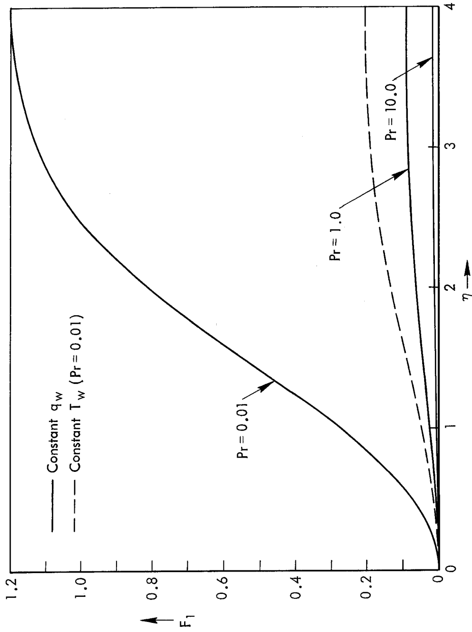
Fig. 4—Function F_1
