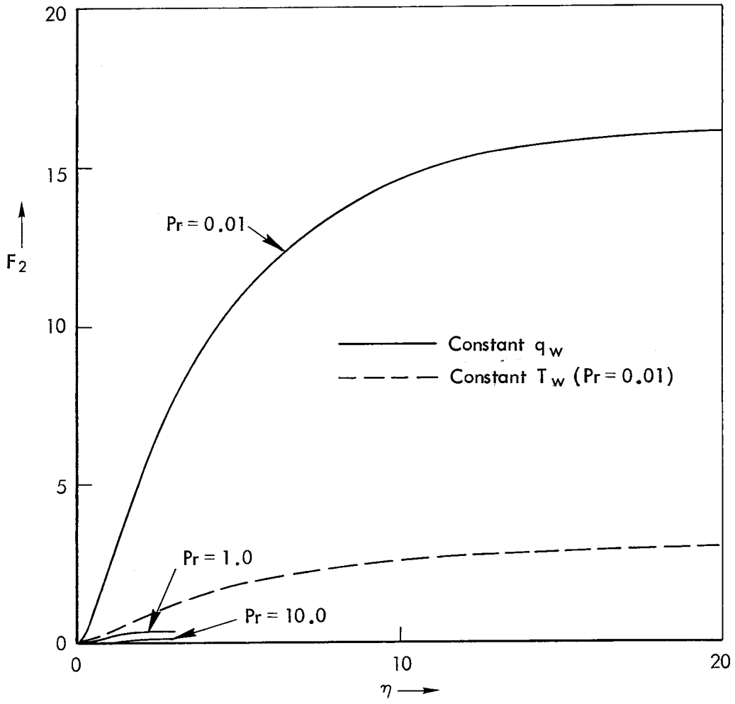
Fig. 6—Function F_2
