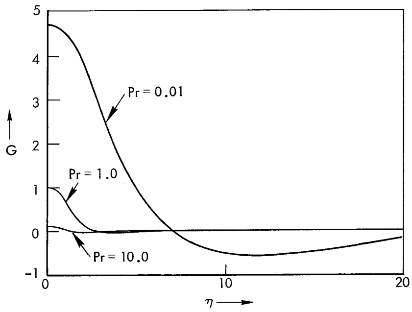
Fig. 3—Function G
