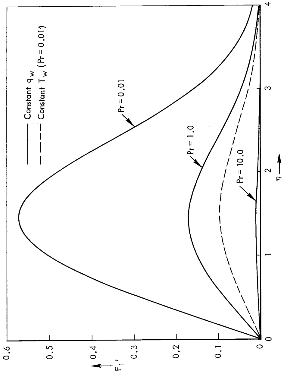
Fig. 5—Function F_1'
