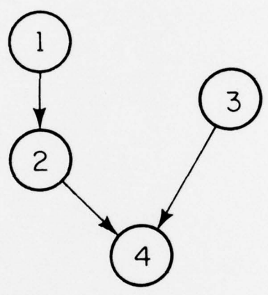
Fig 2.3a PROC
