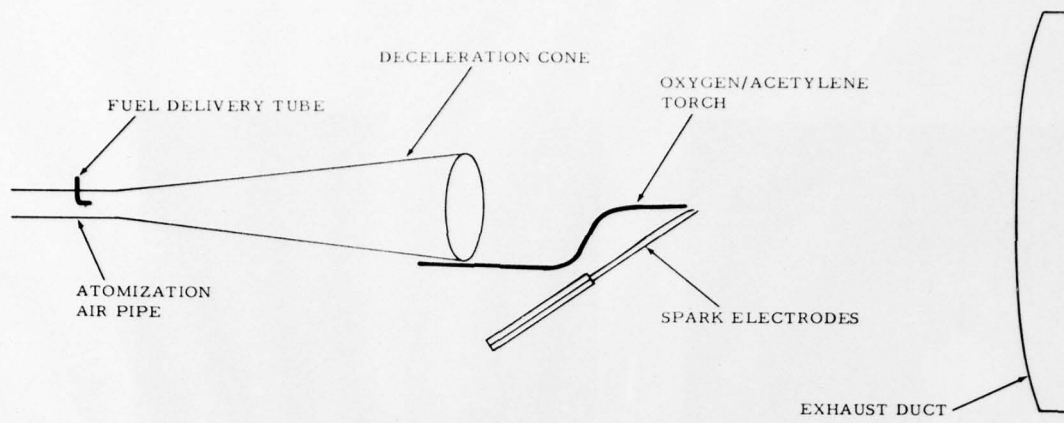
A. TEST SECTION SCHEMATIC
