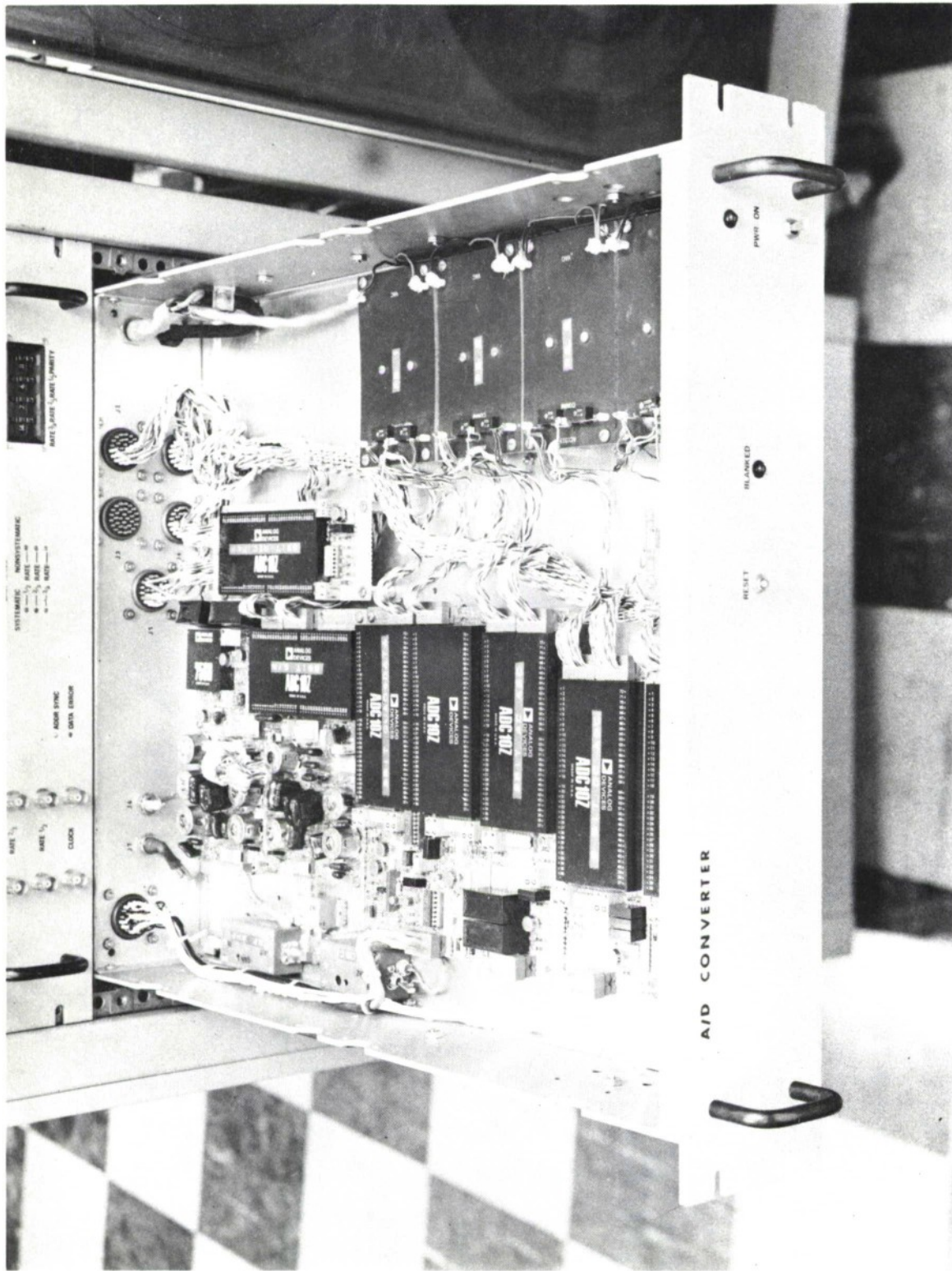
Fig. 25. Analog Drawer.
