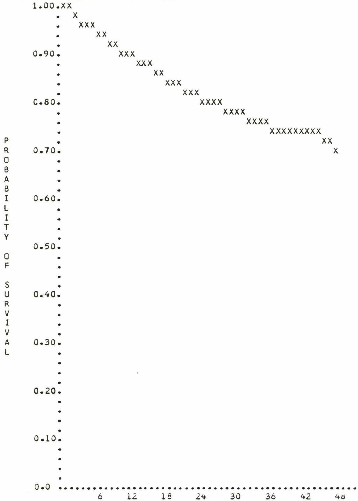
Fig. 7.2—Survival Function
