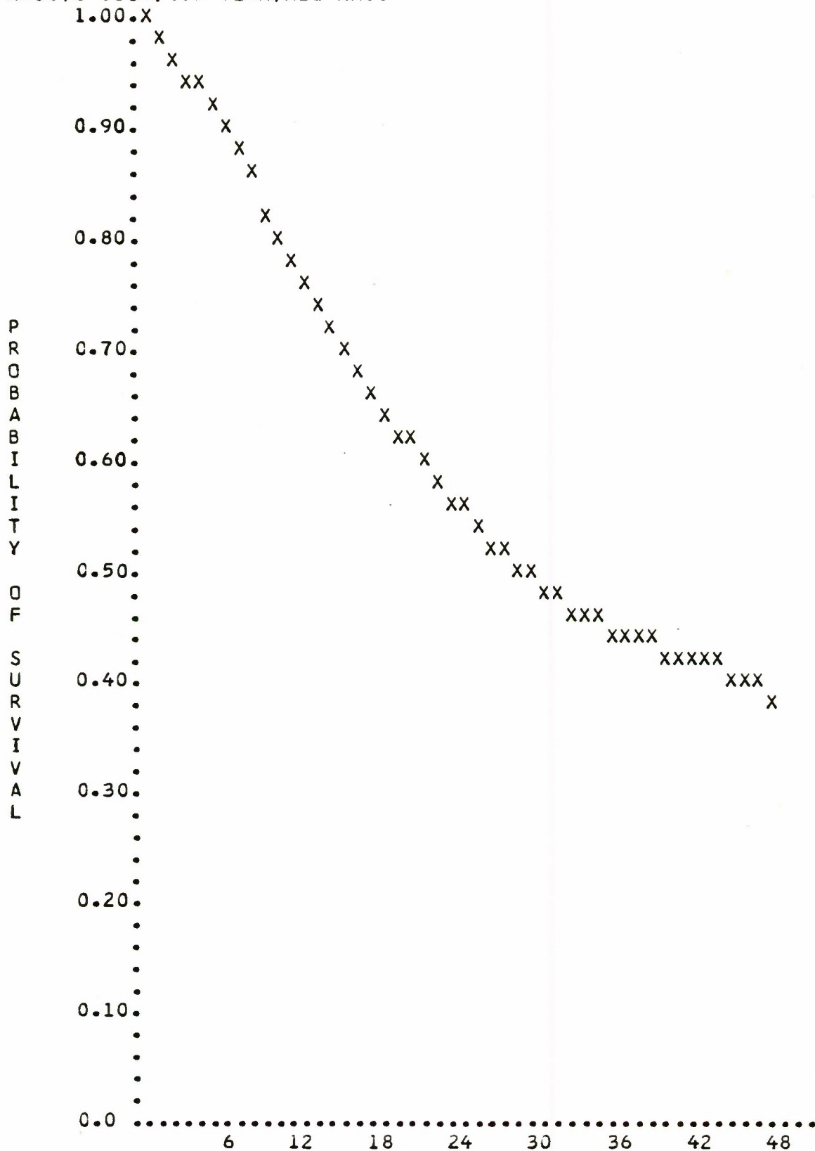
Fig. 7.3— Survival Function
