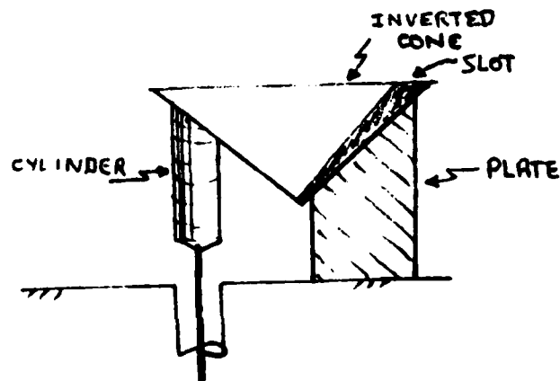
Fig. 4e Broadband Slotted-Cone Antenna
