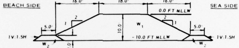
SECTION T-T'
