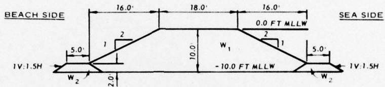
SECTION T-T'
