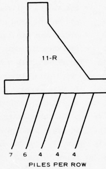
a. Piles battered inward
